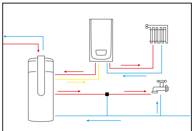
Uproszczony schemat instalacji pompy ciepła z wiszącym kotłem gazowym.
